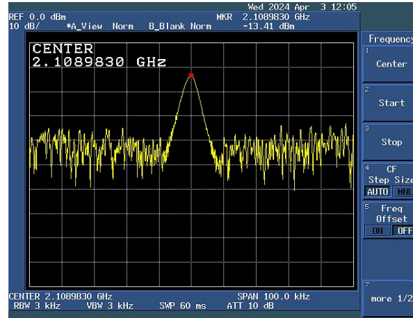
Fig3. 100M CLK module SPAN=100kHz
