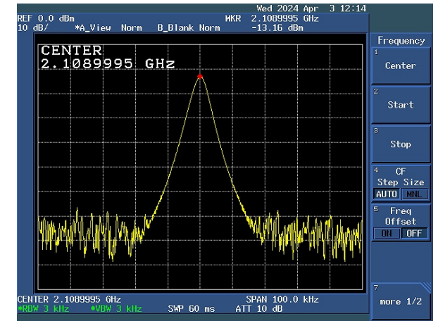
Fig5. 100M OCXO SPAN=100kHz
