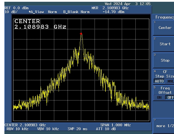
Fig4. 100M CLK module SPAN=1MHz
