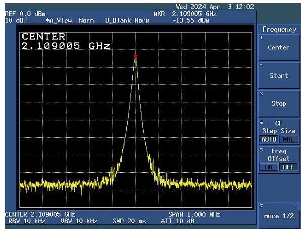
Fig8. 10M OCXO SPAN=1MHz
