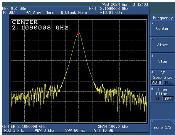
Fig7. 10M OCXO SPAN=100kHz
