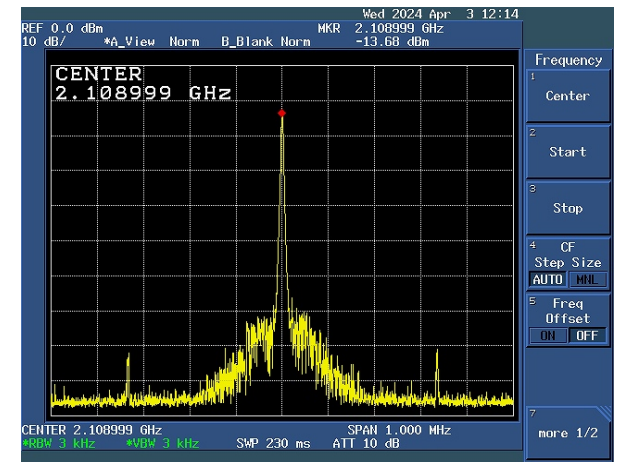
Fig6. 100M OCXO SPAN=1MHz
