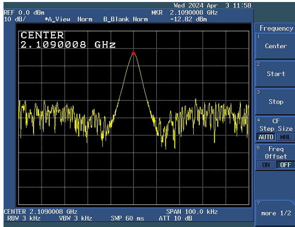
Fig1. 100M TCXO SPAN=100kHz
